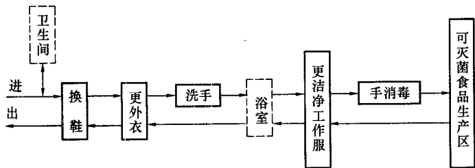
图 5.4.3 可灭菌食品生产区人员净化程序
