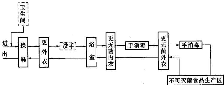
图 5.4.4 不可灭菌食品生产区人员净化程序
