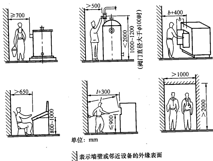
图3 操作设备所需的最小间距
