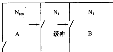
图2 缓冲室门的启闭
