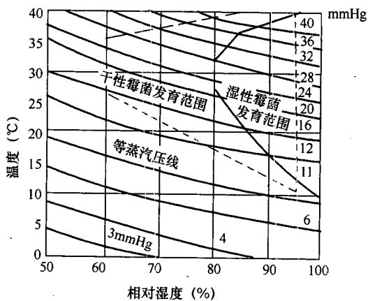
图 4 相对湿度与霉菌的关系
