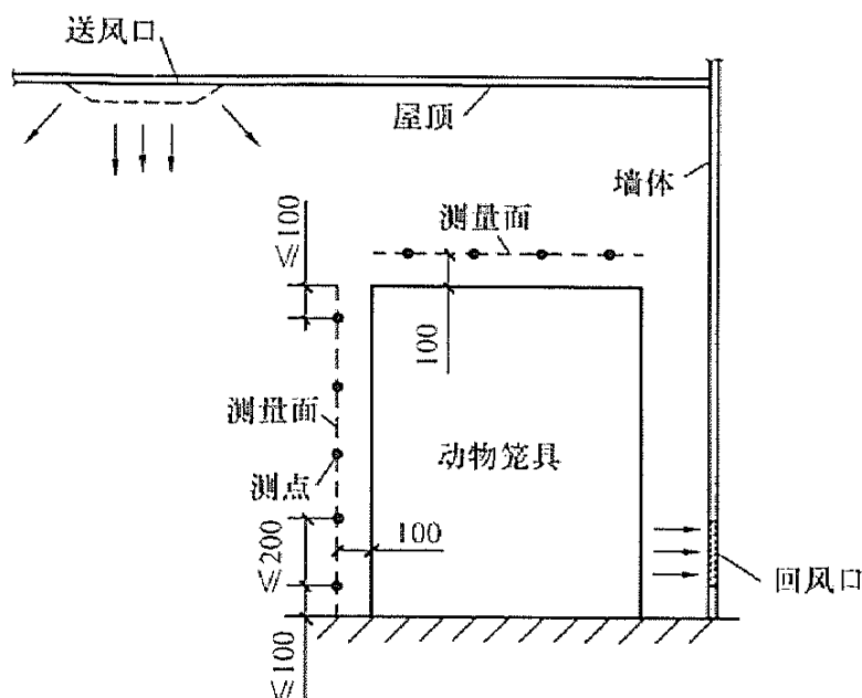
图 10.1.6 测点布置
